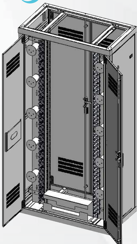
GABINETES PARA ODF ANCHO EXTERNO 90CM 19"
