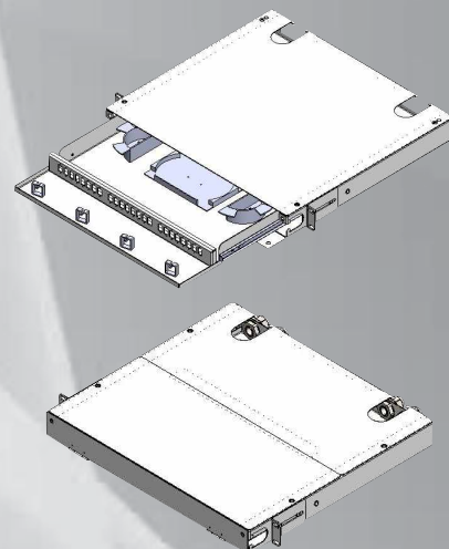
BANDEJAS PARA ODF 19"
