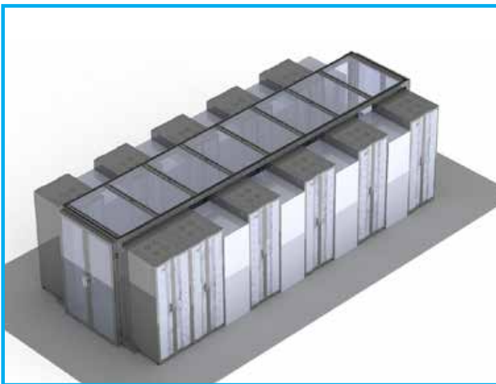
Confinamiento de pasillo frío
